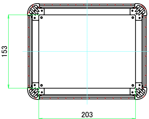
C-C ( 1 : 4.5 )
